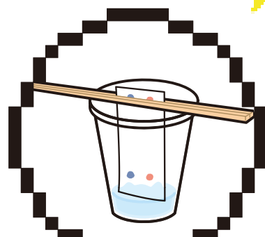
ペーパークロマトグラフィー
